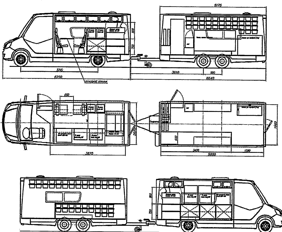
Компоновочная схема
